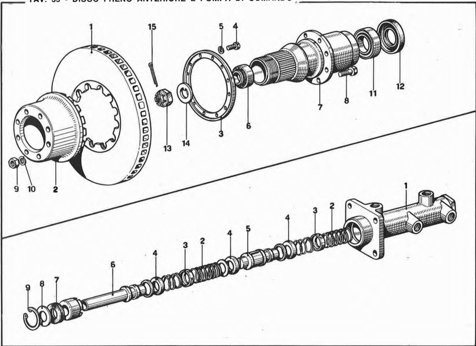
TAV. 35 - DISCO FRENO ANTERIORE E POMPA DI COMANDO
