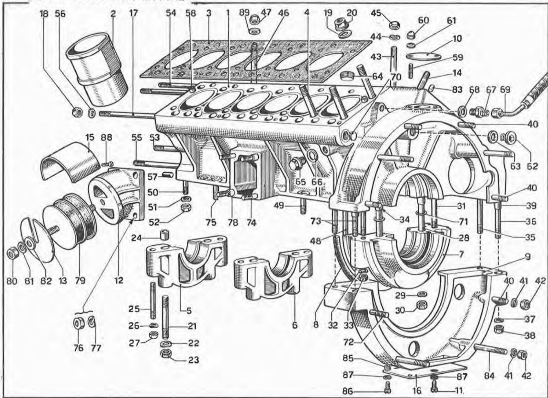
TAV. 1 - BASAMENTO MOTORE
