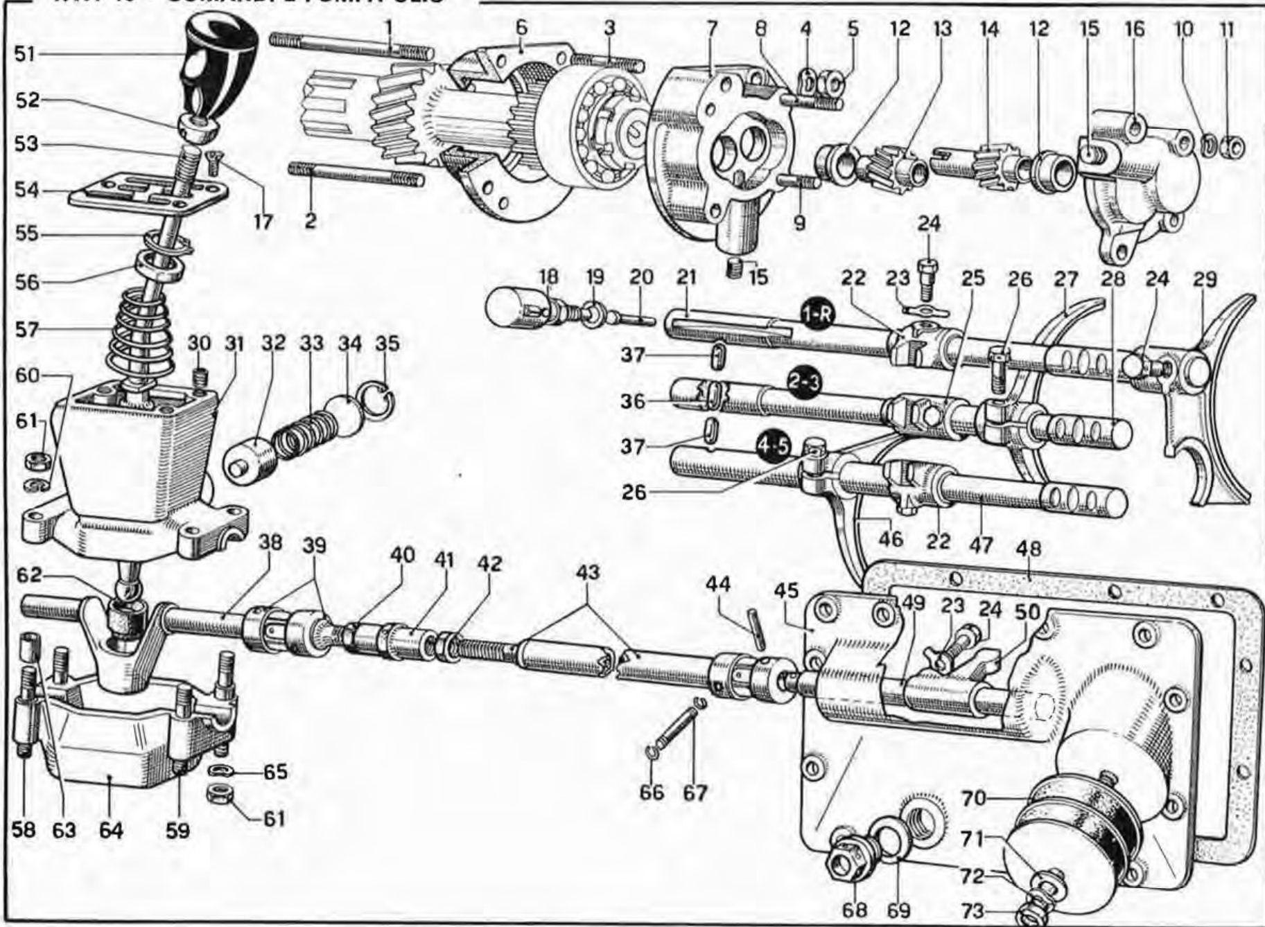
TAV. 19 - COMANDI E POMPA OLIO
