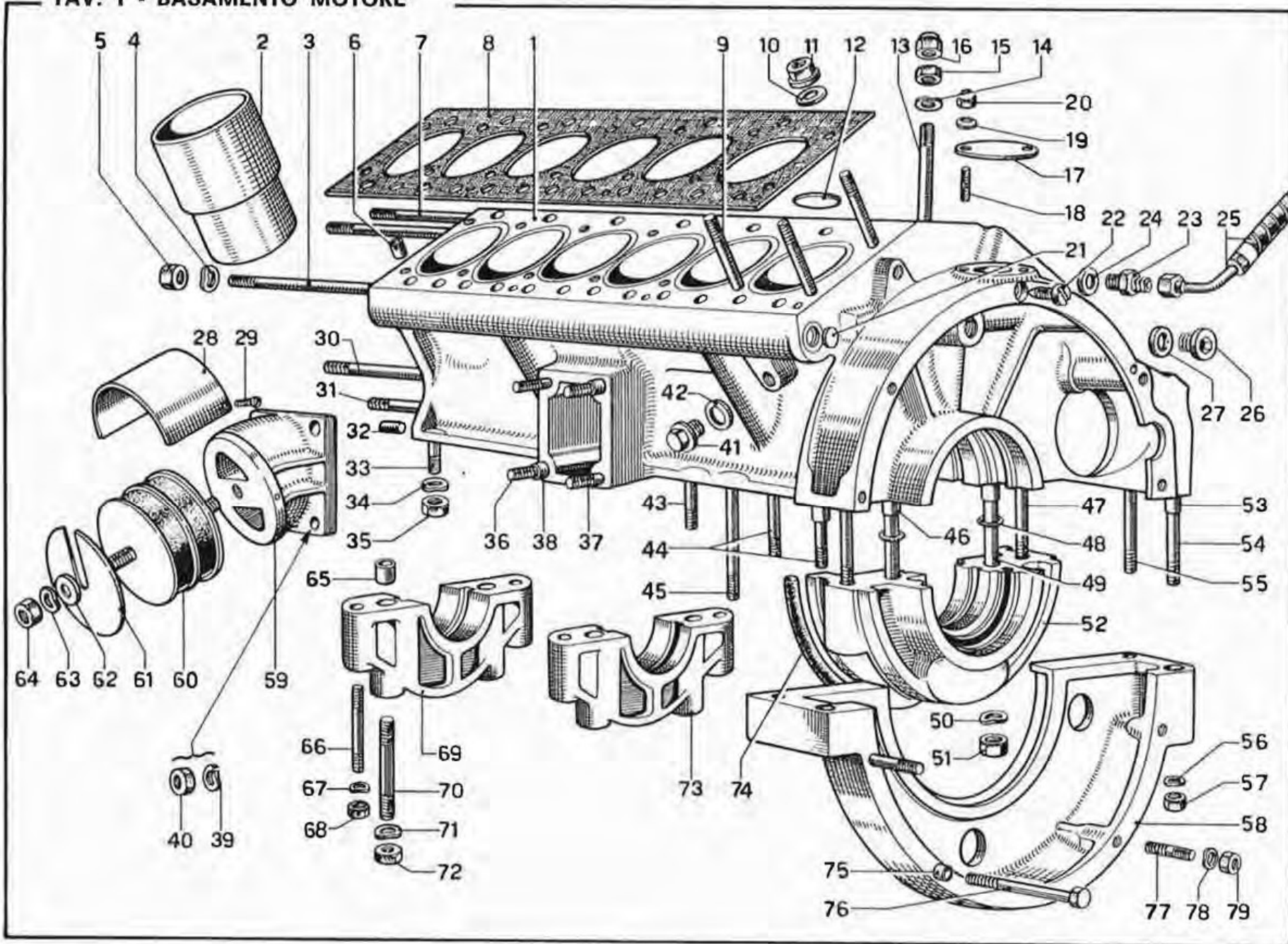
TAV. 1 - BASAMENTO MOTORE
